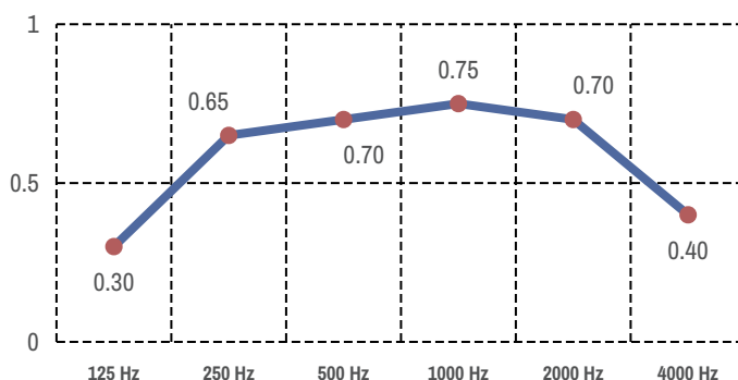
Gráfico de Absorción acústica (NCR e = 15mm)
